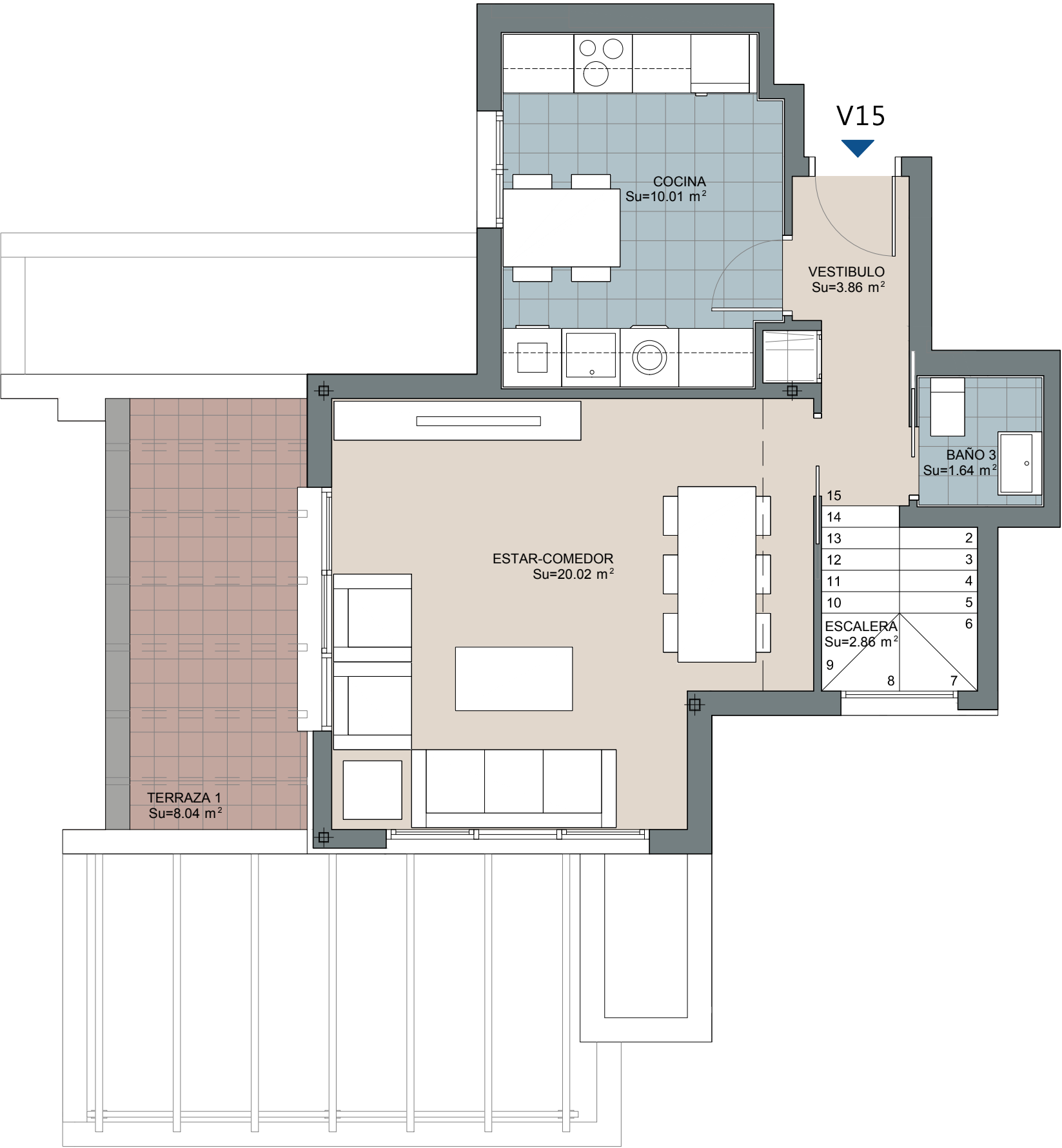
PLANTA ÁTICO
