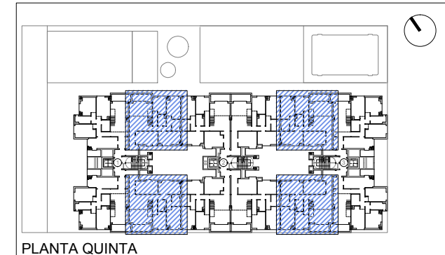
PLANTA QUINTA
