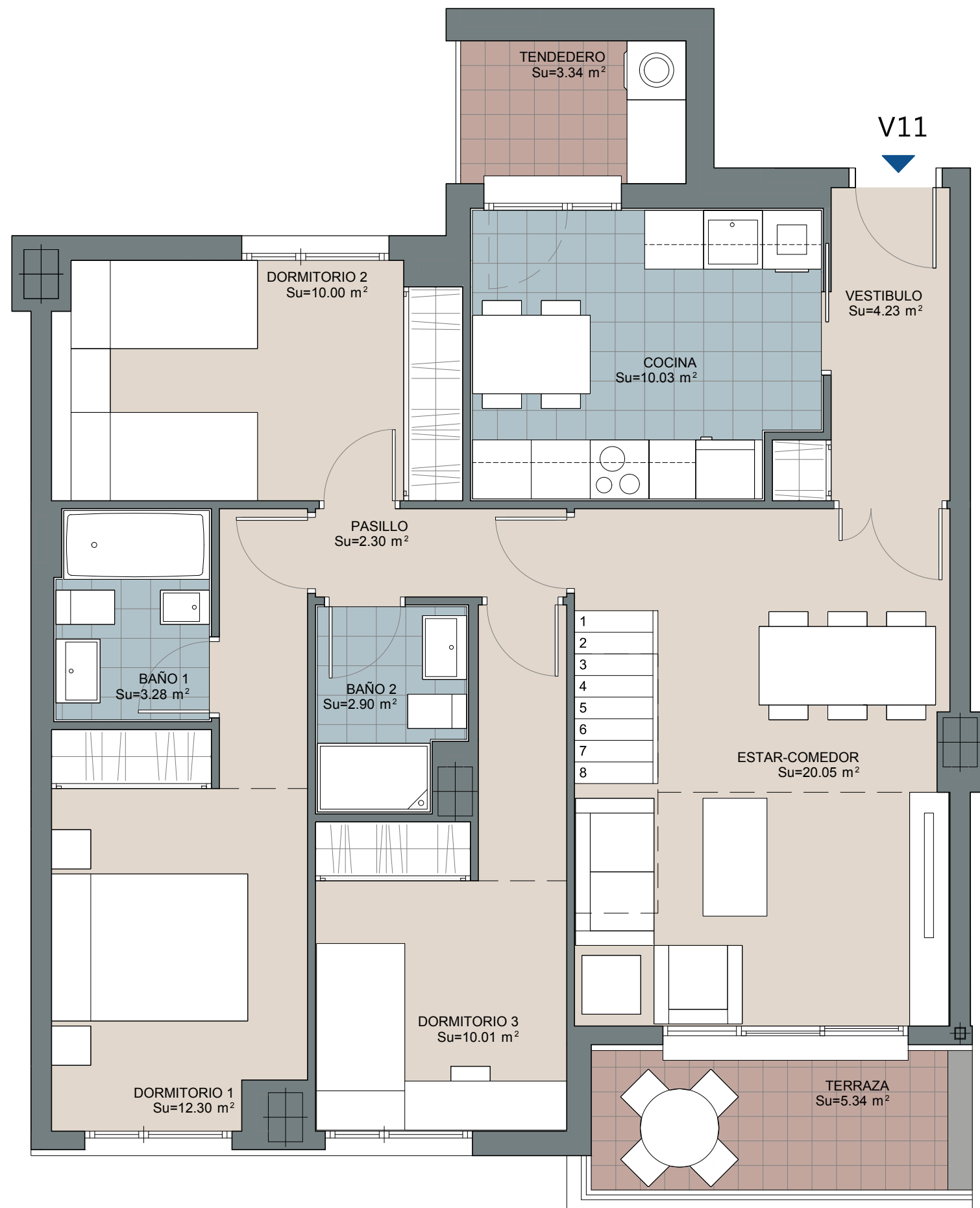
PLANTA QUINTA
