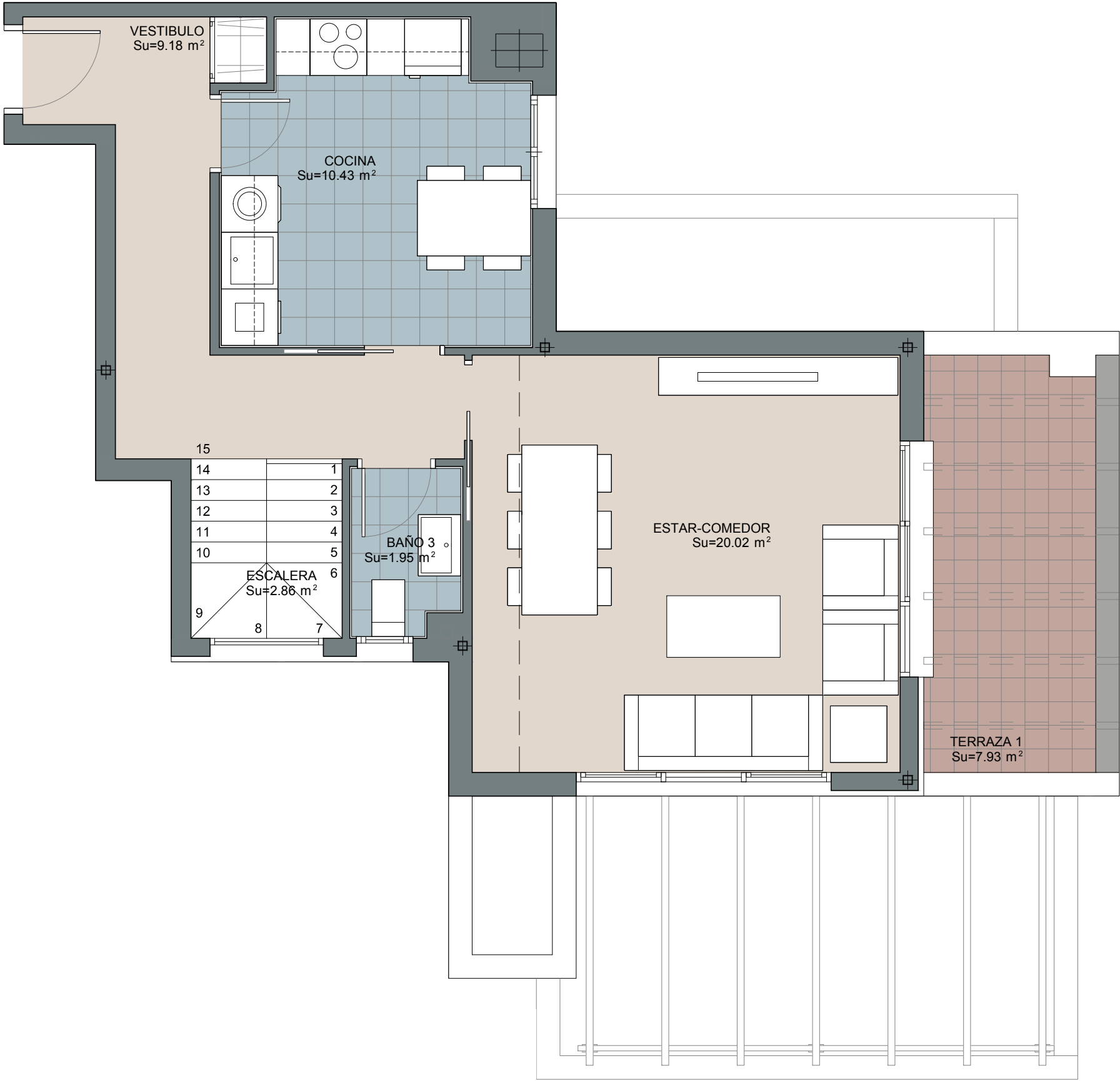
PLANTA ÁTICO
