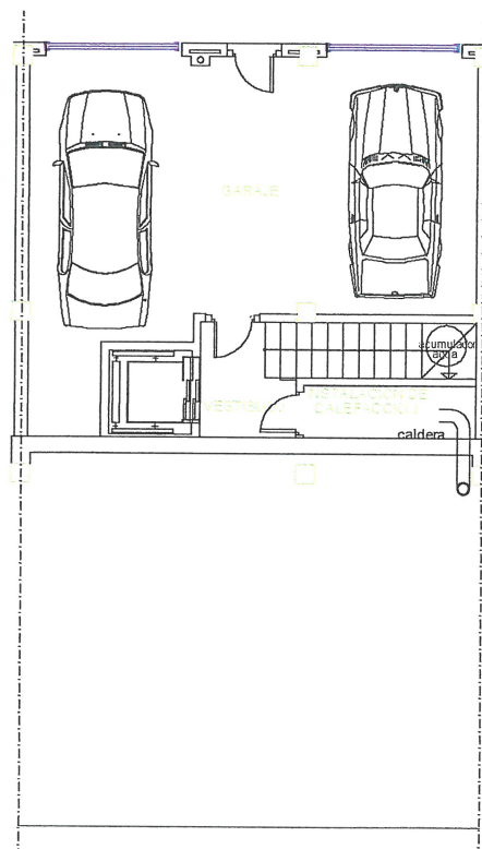
PLANTA DE SOTANO
