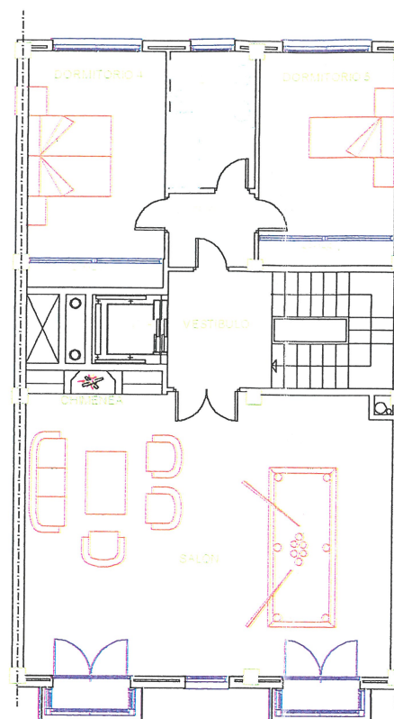
PLANTA SEGUNDA
